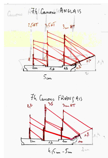
modèles des étais
